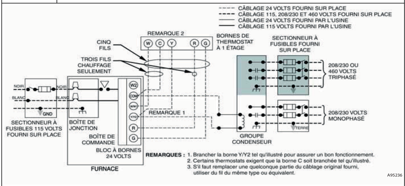
Figure 7 Schéma de câblage du chauffage et de la climatisation – Thermostat à un étage
