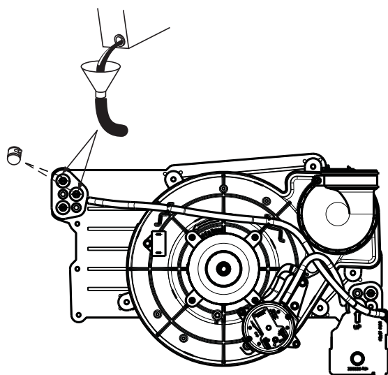
Figure 1 Amorçage du tuyau d'évacuation de condensat
