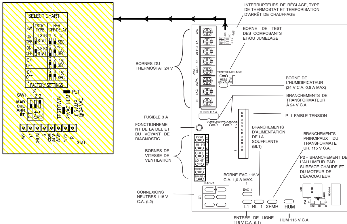
Figure 4 Exemple d'un panneau de commande de chaudière à deux étages
