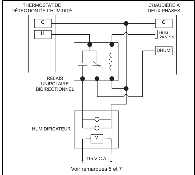
Figure 21 Climatiseur avec chaudière à deux étages, humidificateur et déshumidification
