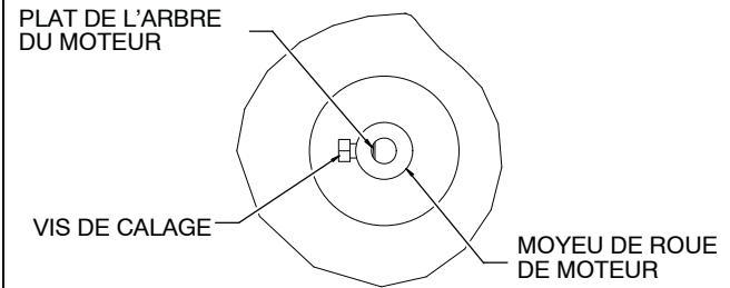
Figure 10 Ensemble de soufflante
