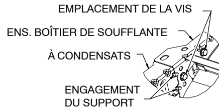
DÉTAIL A
