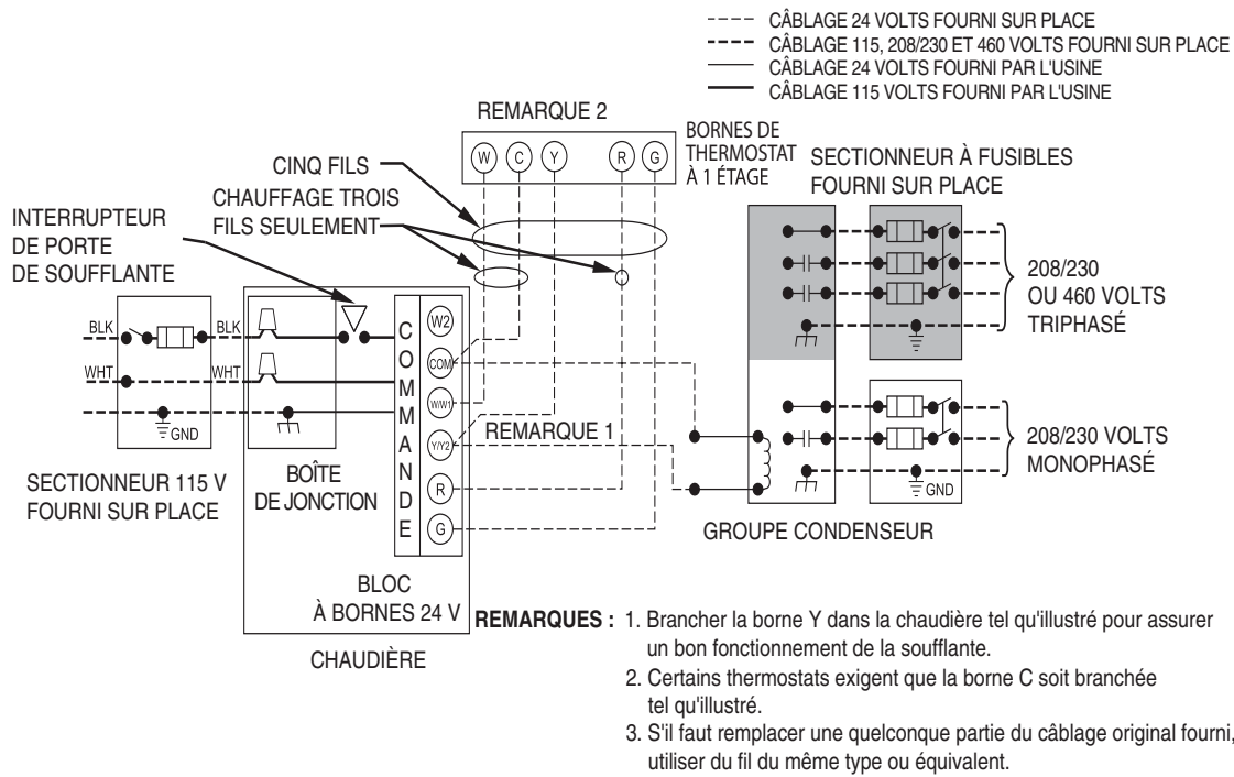
Figure 9 Schéma de câblage du chauffage et de la climatisation – Thermostat à un étage
