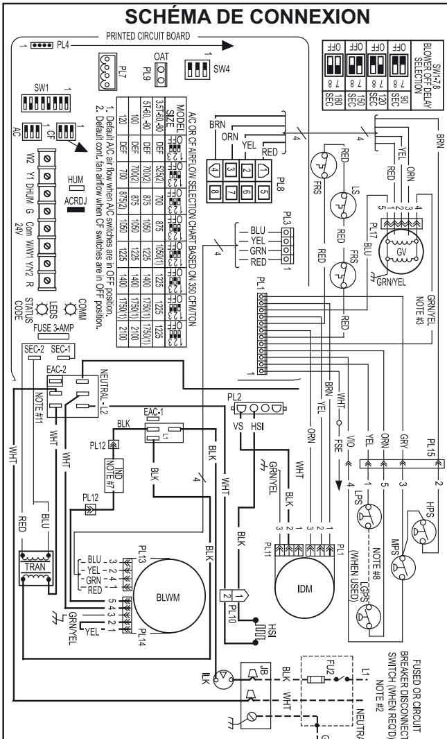
Figure 17 Schéma de câblage
