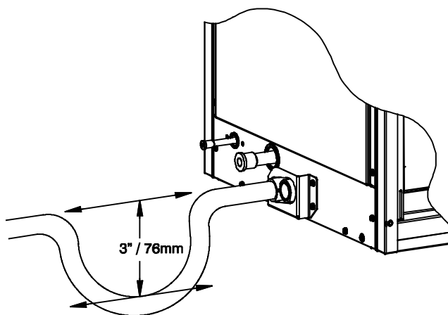
Fig. 3 - Condensate Trap
