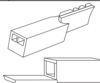
Figure 11 Pose du cavalier de la connexion de gaz propane
