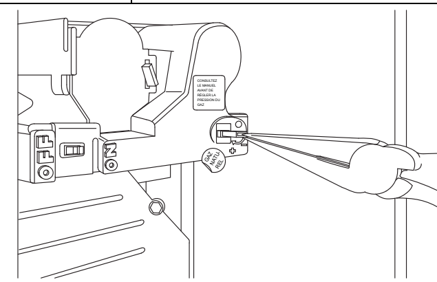
Figure 11 Pose du cavalier de la connexion de gaz propane
