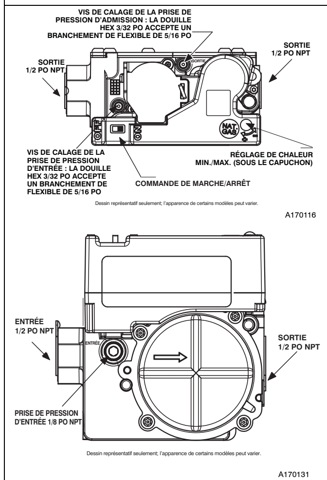
Figure 18 (suite) – (F/G)9MAC et (F/G)9MAE – Distributeur automatique (modulant) sans orifices de pression de tour
