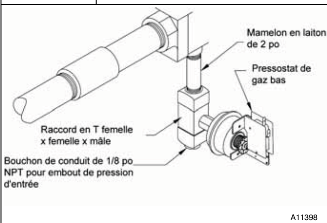
Figure 35 Pressostat de gaz bas 80 %
