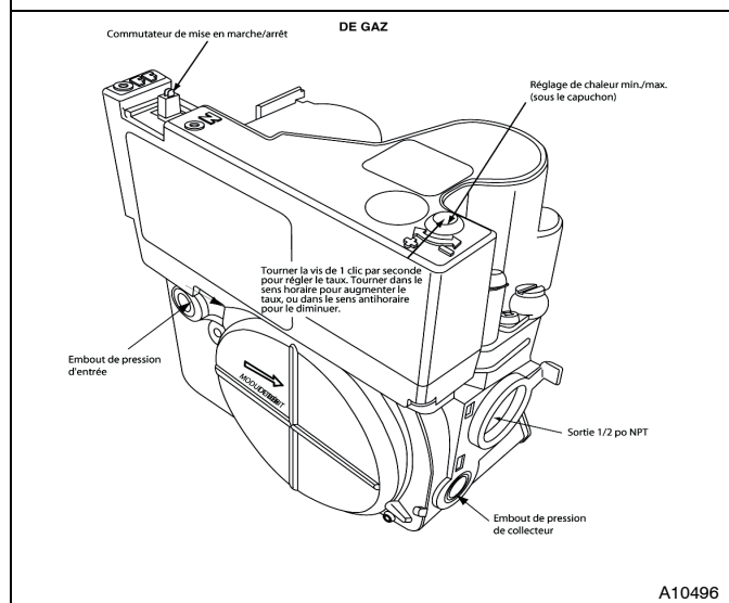
Distributeur automatique (modulant) sans orifices de pression de tour
