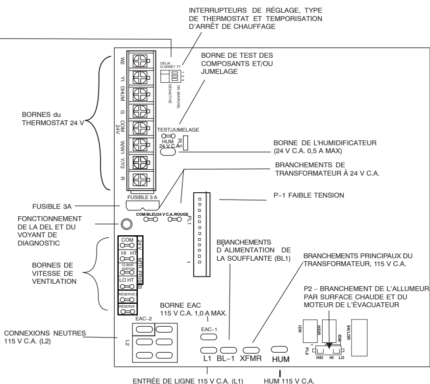
(F/G)9MXT – Exemple de commande de chaudière à deux phases
