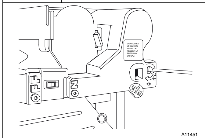
Figure 19 Réglage de la vanne de gaz modulante
