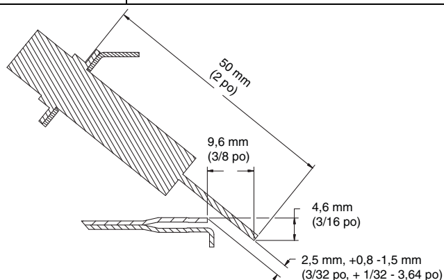
Figure 9 Position de l'allumeur – vue de côté
