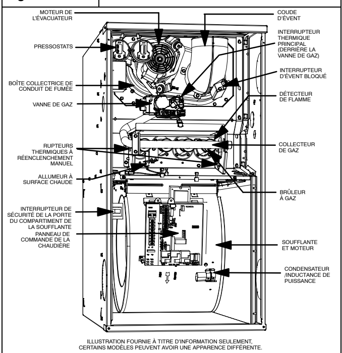
Figure 22 Schéma de la chaudière
