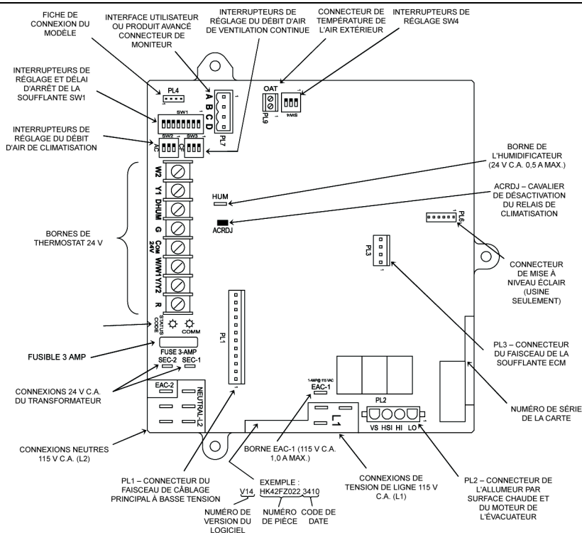
Figure 34 Commande de chaudière – 80 %
