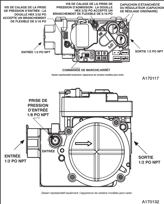
Figure 20 (suite) – Distributeur de gaz automatique (2 phases) avec orifices de pression de tour
