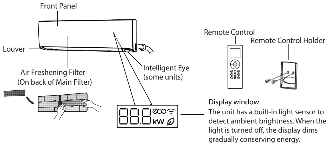
Fig. 1 – Indoor Unit
