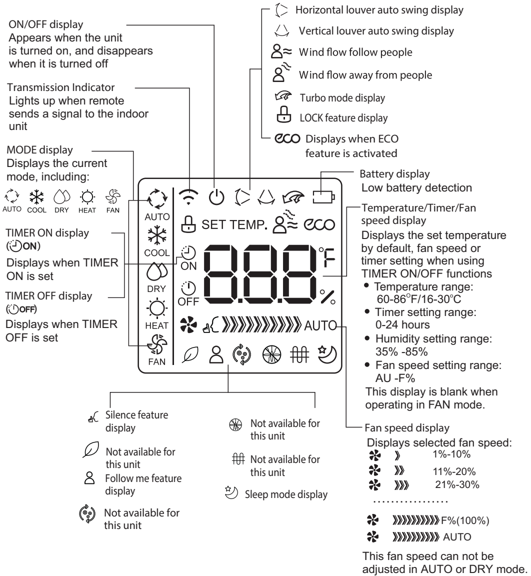
Fig. 4 – Unit Display
