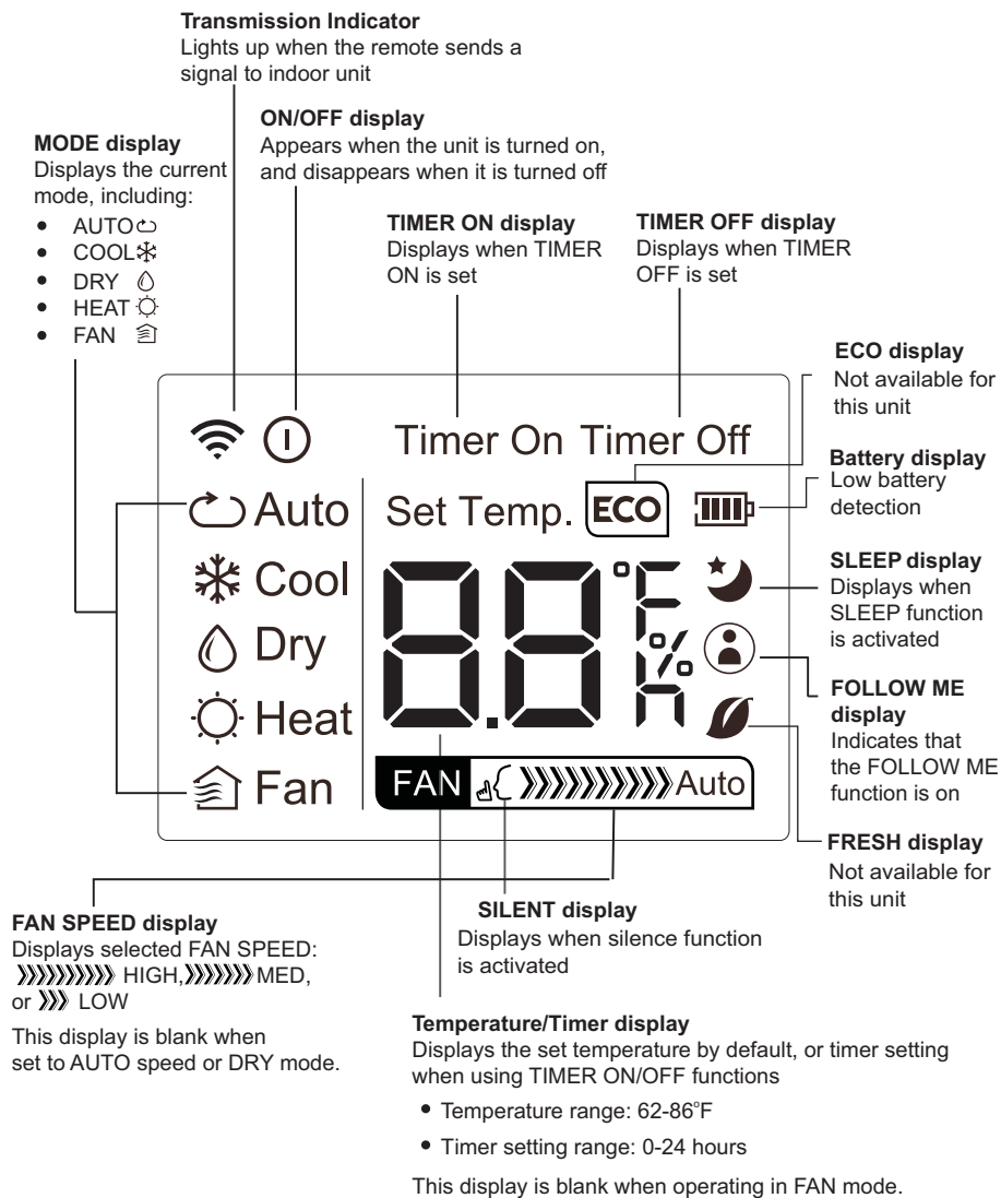
Fig. 5 – Unit Display
